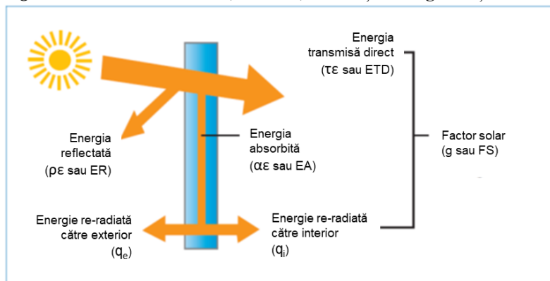
Figura 4. Transmisia, reflexia, absorbția energetică și factorul solar
