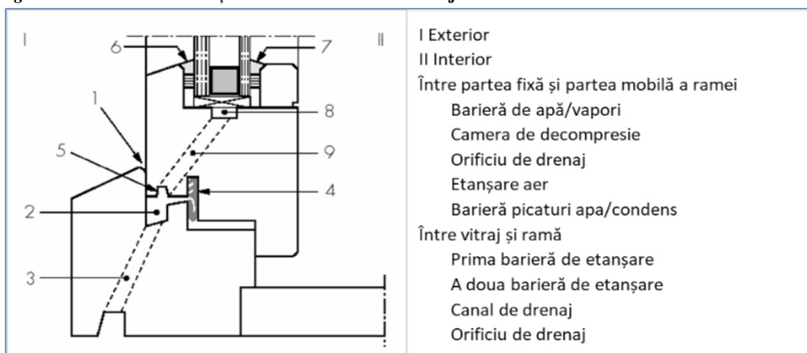
Figura 10. Schema secțiune transversala ramă-vitraj
