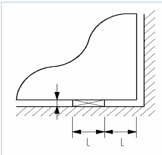
Figura 12. Poziționarea calelor față de colțul vitrajului
