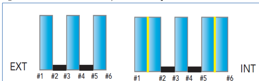
Figura 1. Numerotarea fețelor unui vitraj izolat
